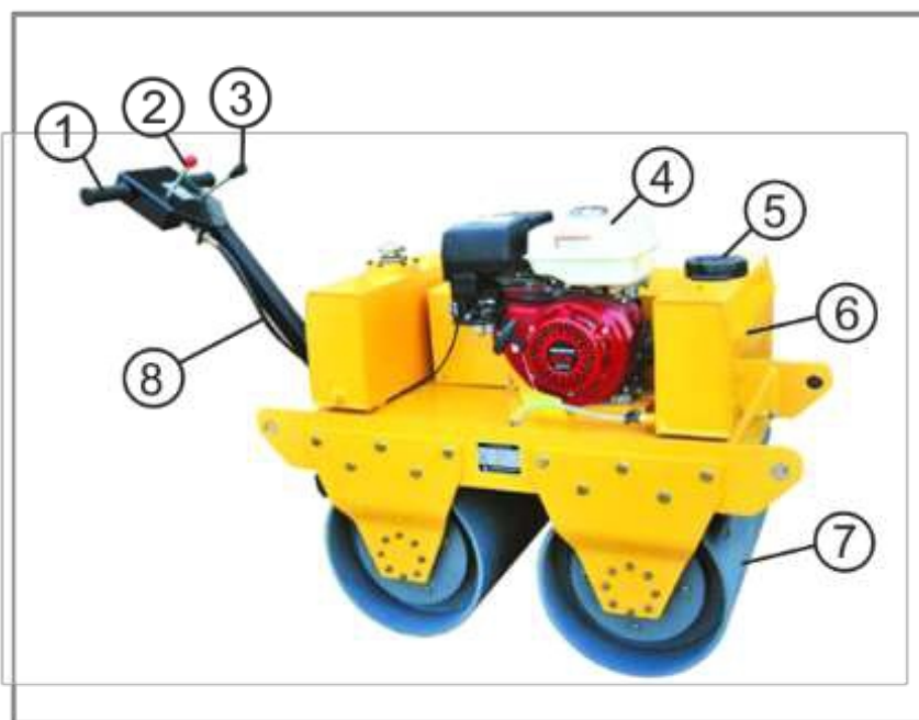
VRDR-600 (двухвальцовый)
