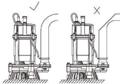
(Насос с гибкой трубой)
